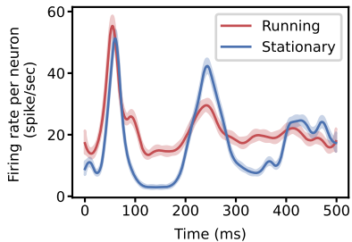
V1
